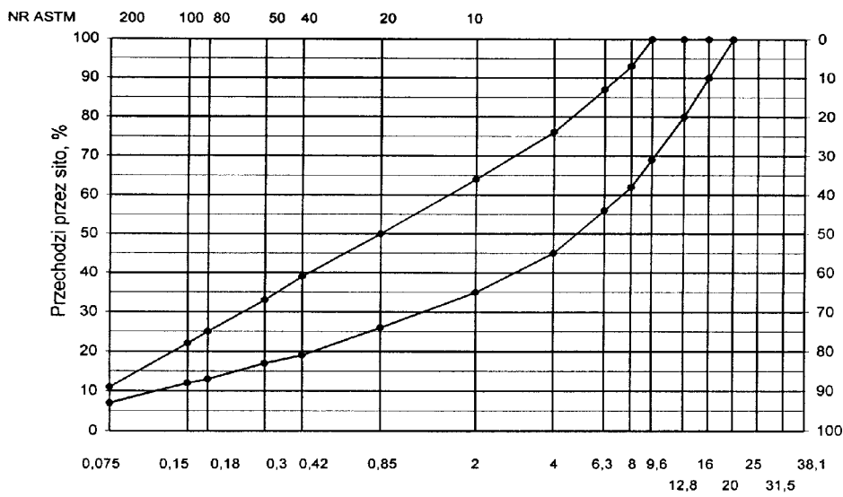
Rys. 2. Krzywe graniczne uziarnienia a mieszanki mineralnej BA od 0 do 16mm, od 0 do 12,8 mm do warstwy ścieralnej nawierzchni drogi o obciążeniu u ruchu KR1 lub KR2
