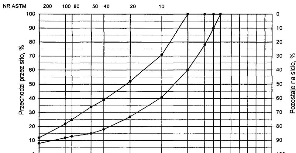
Rys. 3. Krzywe graniczne uziarnienia mieszanki mineralnej BA od 0 do 8mm, od 0 do 6,3 mm do warstwy ścieralnej nawierzchni drogi o obciążeniu ruchu nawierzchni drogi o obciążeniu ruchu KR1 lub KR2
