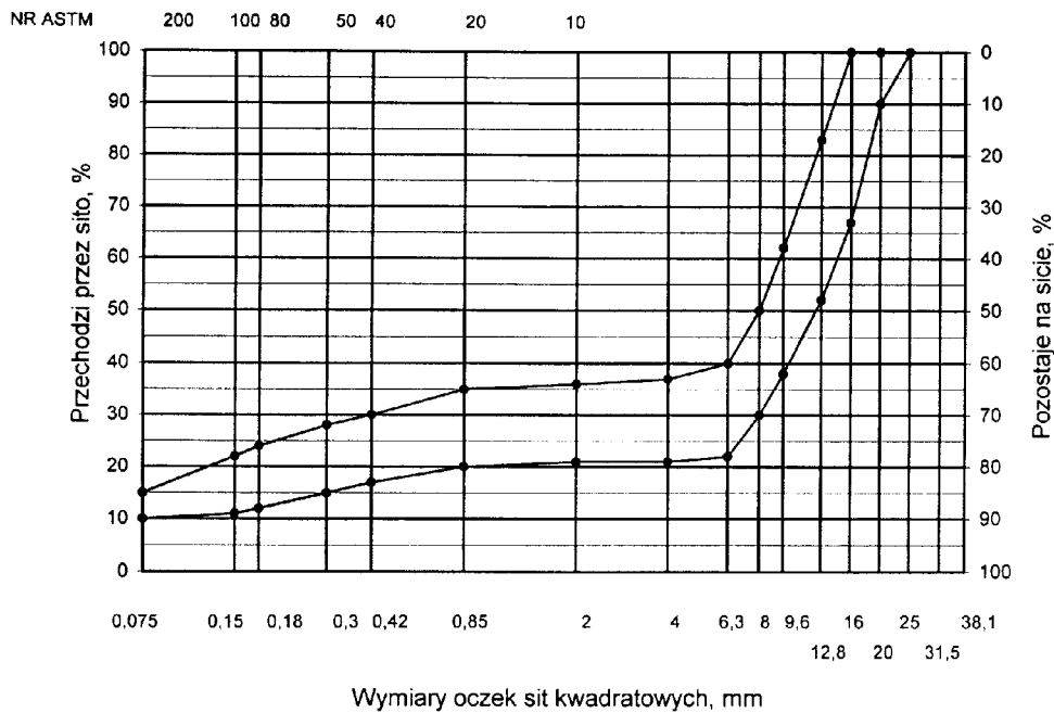
Rys. 5. Krzywe graniczne uziarnienia a mieszanki mineralnej BA od 0 do 20 mm (mieszanka o nieciągłym uziarnieniu) do warstwy ścieralnej nawierzchni drogi o obciążeniu w ruchu od KR3
