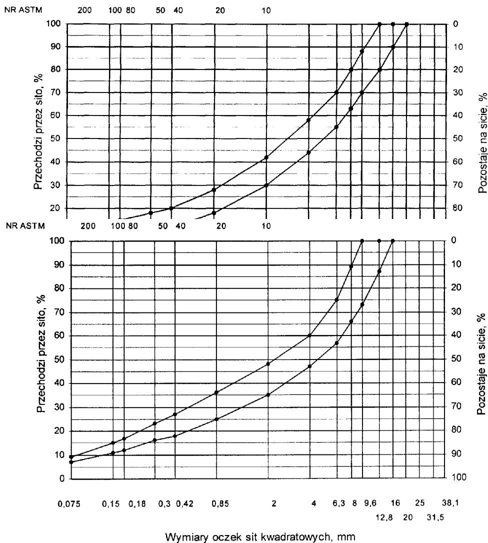
Rys. 6. Krzywe graniczne uziarnienia mieszanki mineralnej BA od 0 do 16 mm do warstwy ścieralnej nawierzchni drogi o obciążeniu w ruchu od KR3 do KR6
