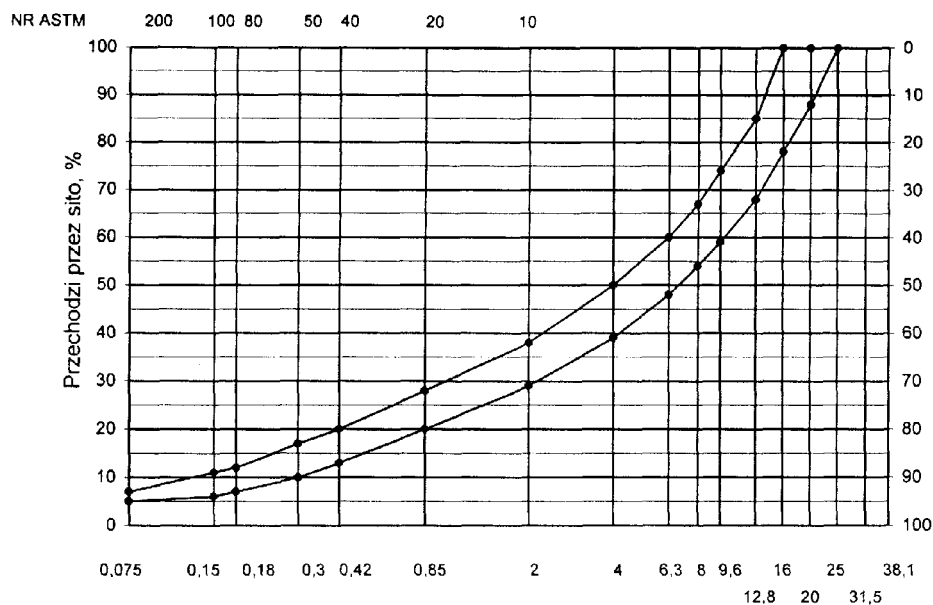
Rys. 4. Krzywe graniczne uziarnienia mieszanki mineralnej BA od 0 do 20 mm do warstwy ścieralnej nawierzchni drogi o obciążeniu ruchu od KR3 do KR6
